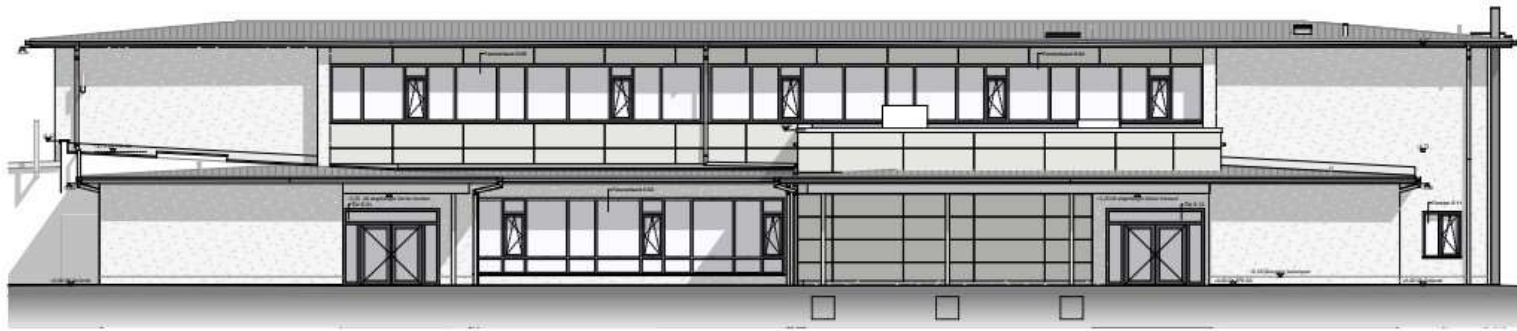
ANSICHT NORD-WEST
