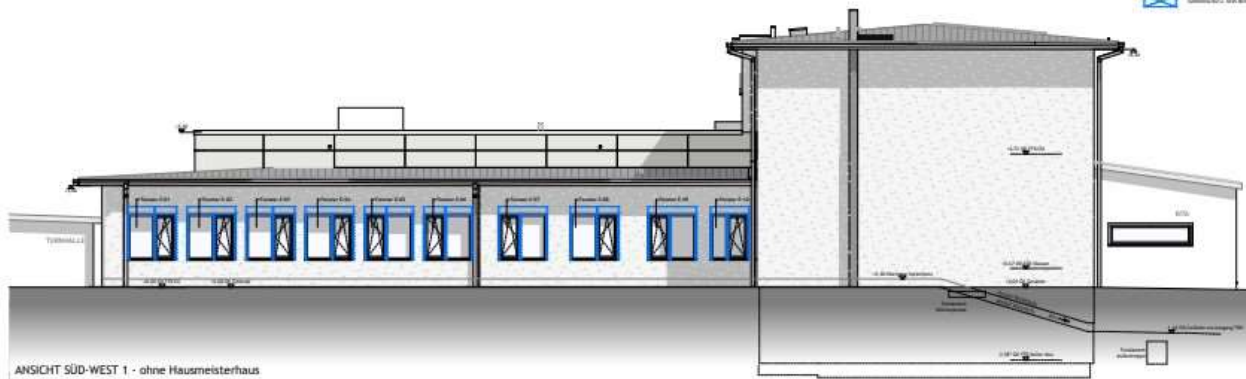
ANSICHT SÜD-WEST 1 - ohne Hausmeisterhaus
